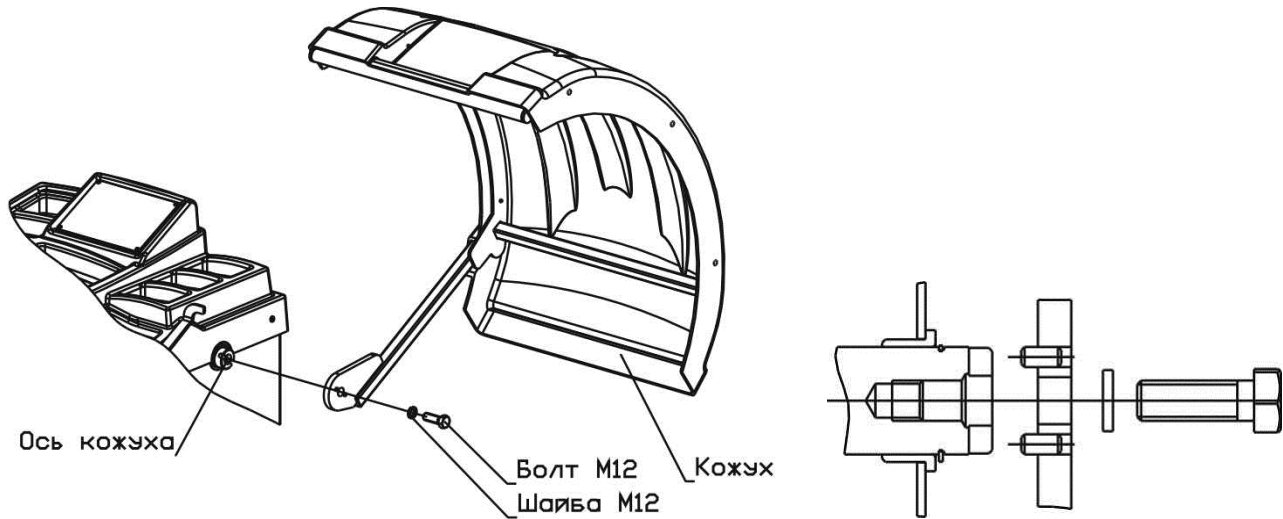
Рисунок 4.7 – Монтаж кожуха
